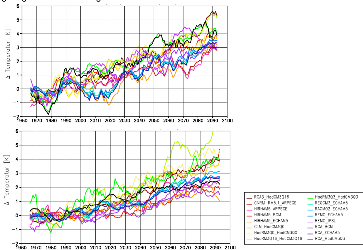
Abbildung 3.4: Projizierte Änderung der 2 m-Temperatur [K] im A1B-Szenario simuliert mit 16 Global-/Regionalmodell-Kombinationen in Winter (oben) und Sommer (unten) im Gebietsmittel Deutschland relativ zu 1971-2000 (gleitendes 11-Jahresmittel)
